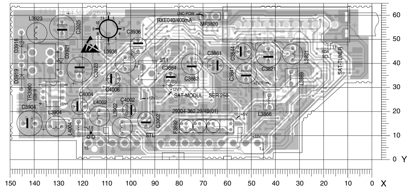
Côte composants, Vue de dessus / Component Side, Top View
